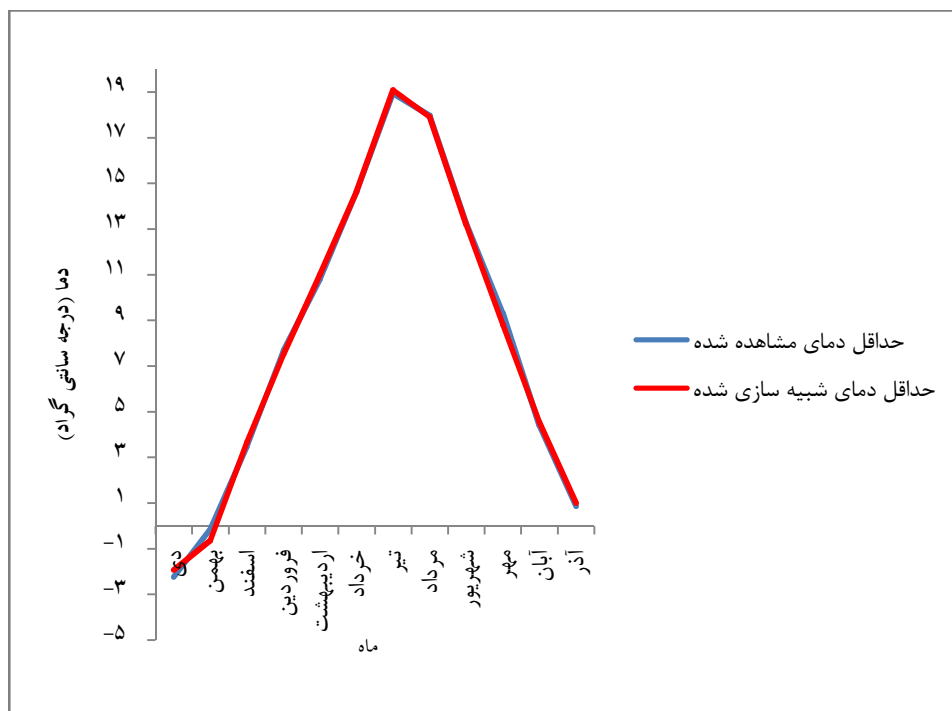
شکل ۴: دمایی حدافل مشاهده شده و شبیه سازی شده ایستگاه انتخابی حوضه بختیاری توسط مدل لارس طی دوره آماری ۱۹۸۹-۲۰۰۸
