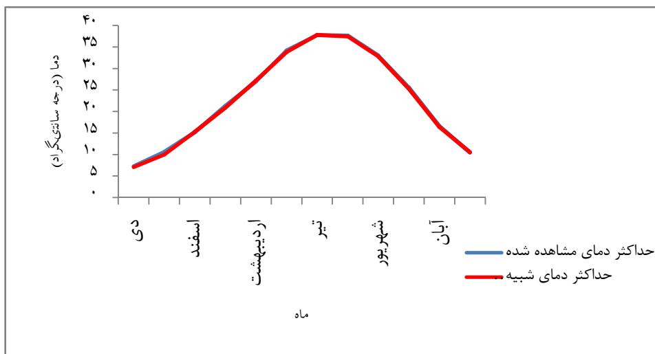
شکل ۵: دمایی حداکثر مشاهده شده و شبیه سازی شده ایستگاه انتخابی حوضه بختیاری توسط مدل لارس طی دوره آماری ۱۹۸۹-۲۰۰۸
