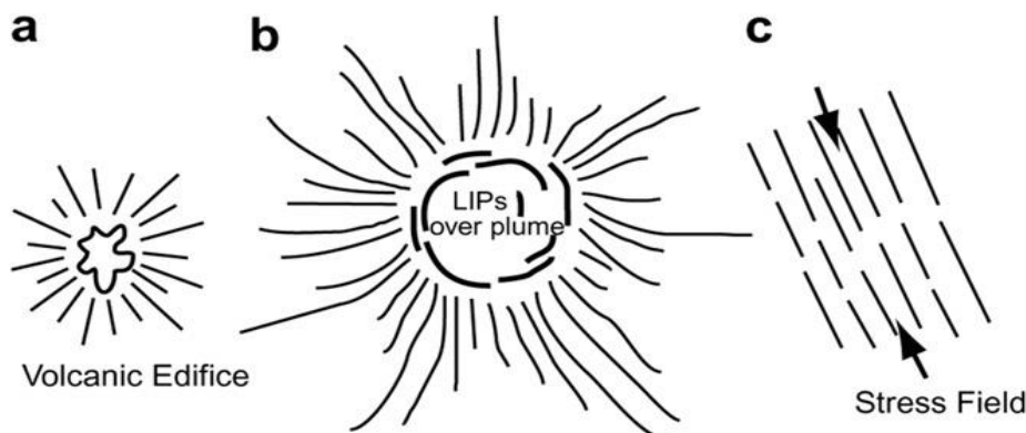
شکل ۲. تقسیم بندی انواع دایک فوجی منبع: (Hou, 2012: 6).
