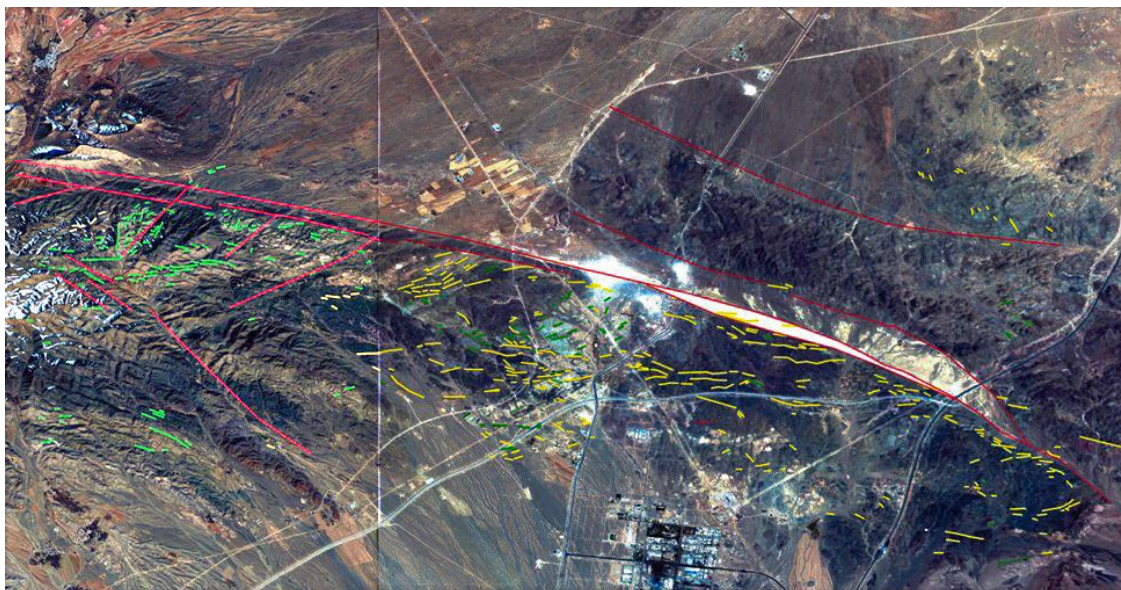
شکل ۳. دایک‌های شمال ساوه بر تصویر ماهواره ای منبع: (بازوبندی، ۱۳۹۴: ۱۶۸)
