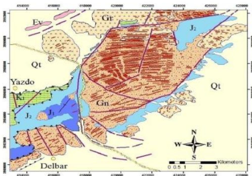
شکل ۴. دایک‌های فوجی دلبر بر نقشه زمین‌شناسی منطقه منبع: (اصغرزاده، ۱۳۹۲: ۱۷۸).
